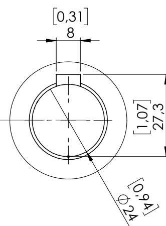
SEZIONE A-A
